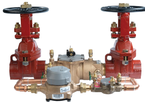
007M1DCDA-OSY con sensor de congelación
