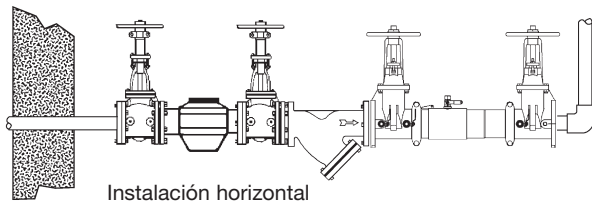
Instalación horizontal
