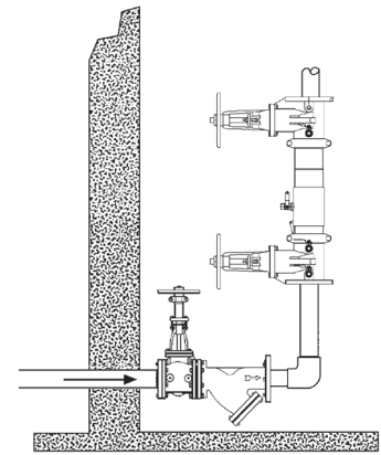
Instalación vertical
