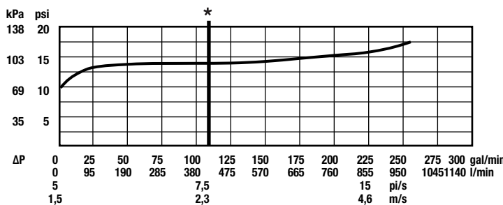
2 ½ po (6,4 cm)
