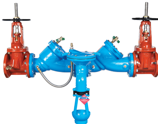
LF909 avec capteur d'inondation et lame d'air
