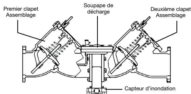
LF909 avec capteur d'inondation et lame d'air
