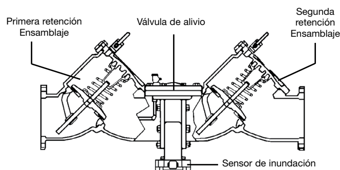
LF909 con sensor de inundación y espacio de aire
