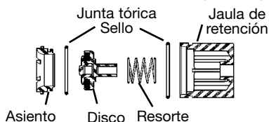
CONJUNTO DE RETENCIÓN \frac{3}{4} " (1.90 cm) M3
