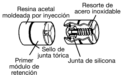
CONJUNTO DE RETENCIÓN DE \frac{1}{4} " – \frac{3}{4} " (0.64 cm - 1.90 cm)
