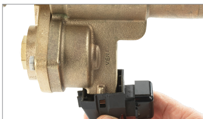
2. Enfoncez le capteur sur la soupape de décharge.
